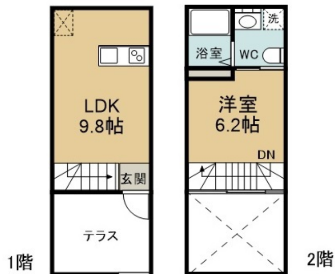
【間取り図】
